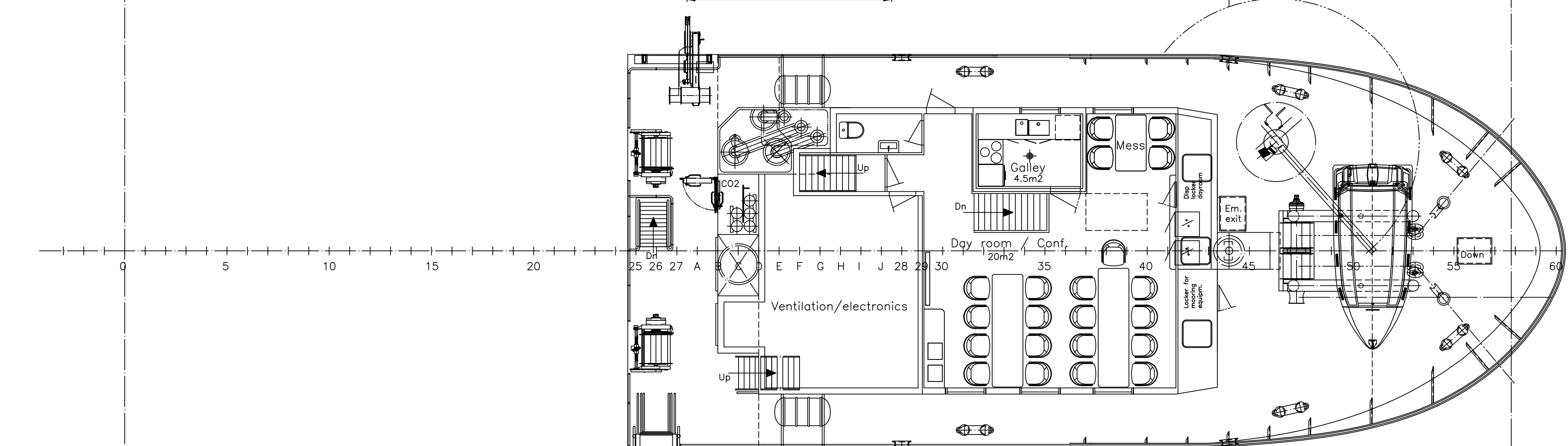
A-DECK
