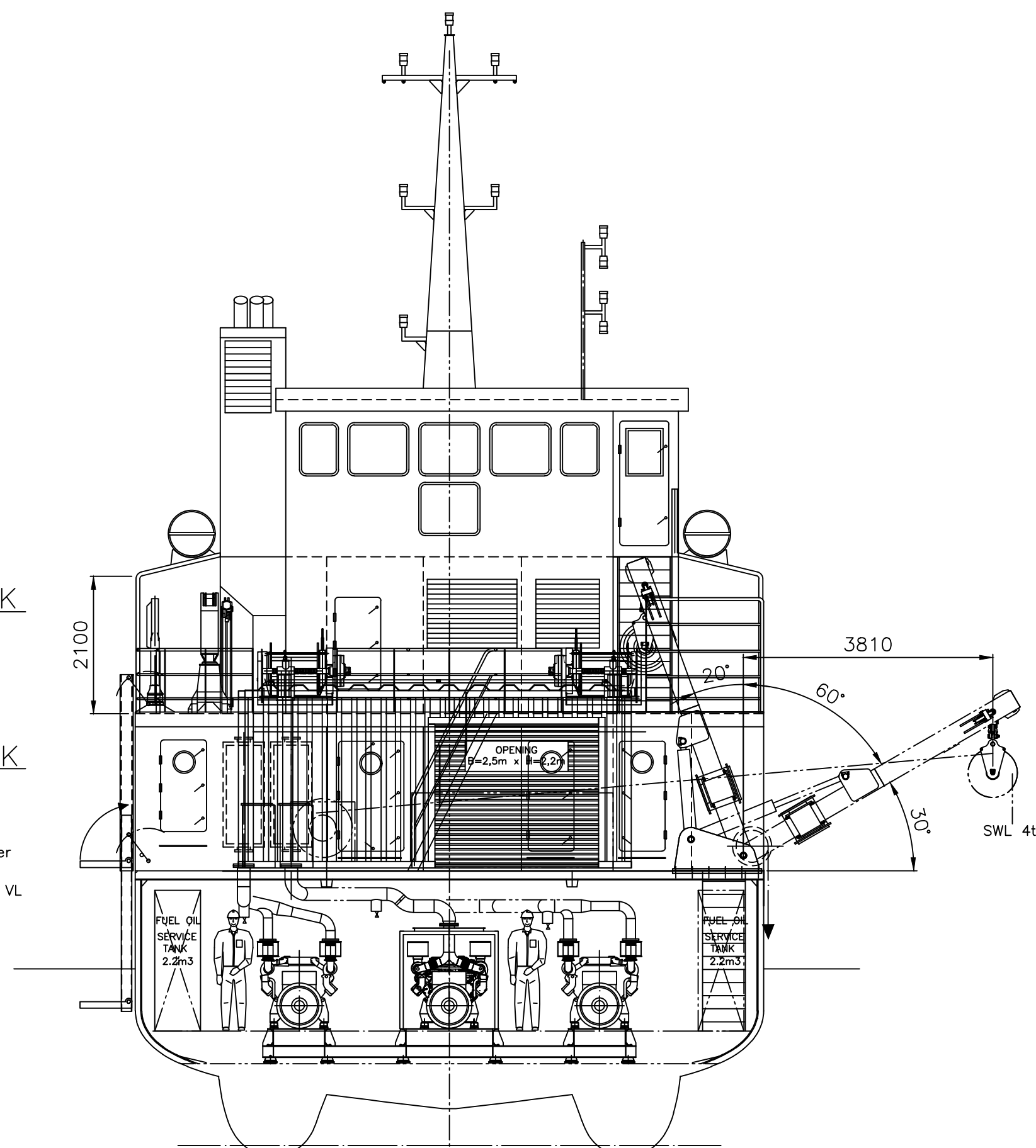
SECTION FR.17
